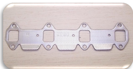
Articolo 7076 Guarnizione per attacco collettore su motori Chrysler M80.
